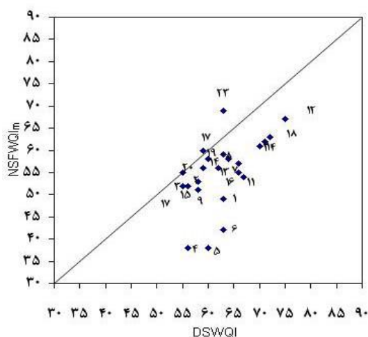
شکل ۴- مقایسه شاخص های کیفی DS WQI و NSFQI m در ایستگاههای انتخابی سد کرخه
