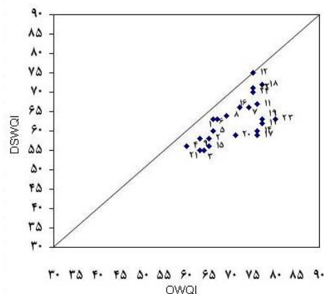
شکل ۱- مقایسه شاخص های کیفی DS WQI و OWQI در ایستگاههای انتخابی سد کرخه
