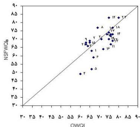
شکل ۲- مقایسه شاخص های کیفی NSF QI a و OWQI
